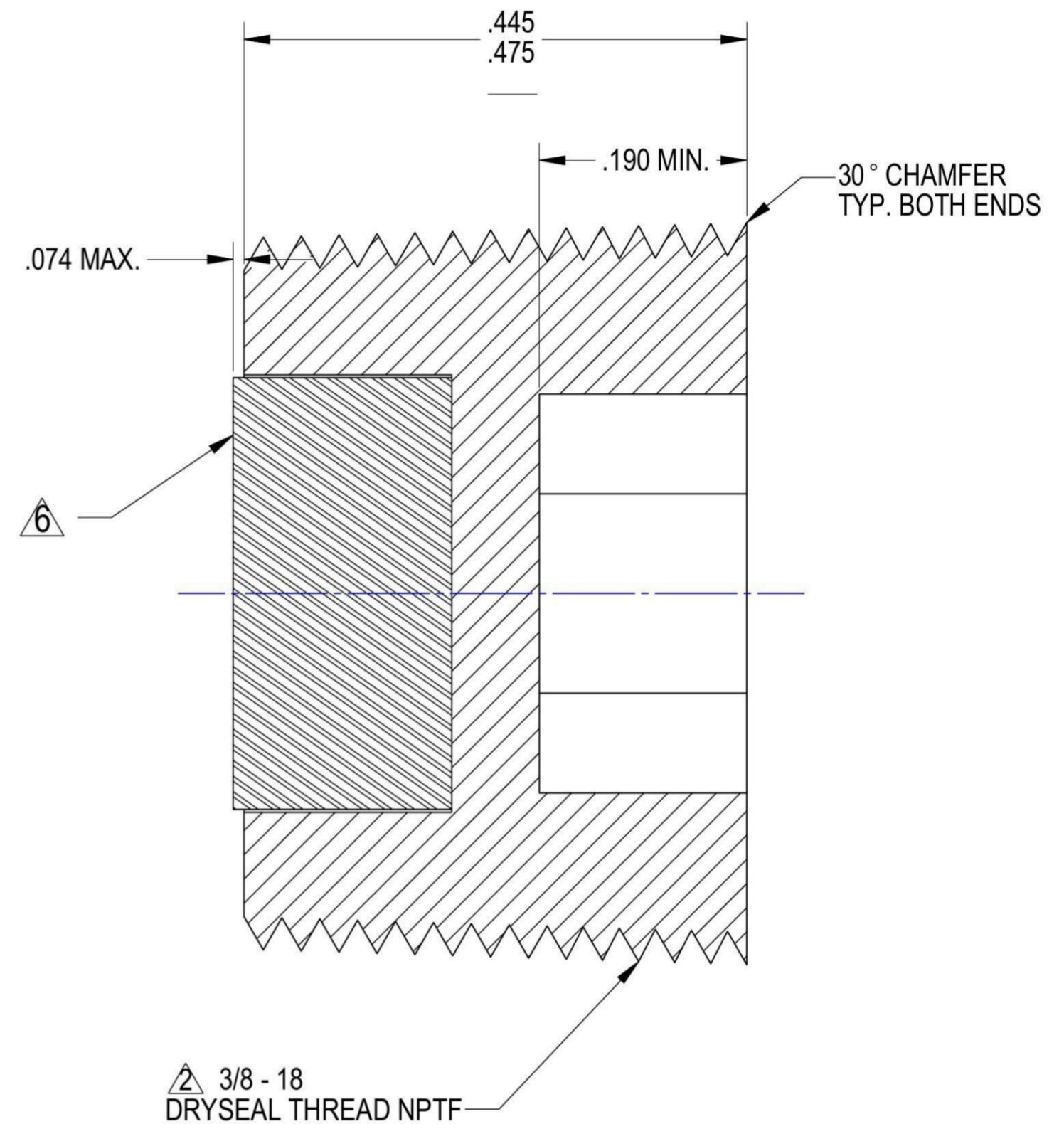
SECTION A-A
